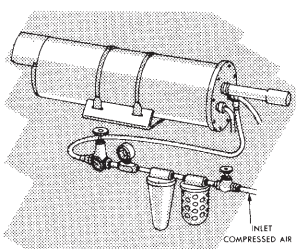
産業用テレビカメラの冷却
